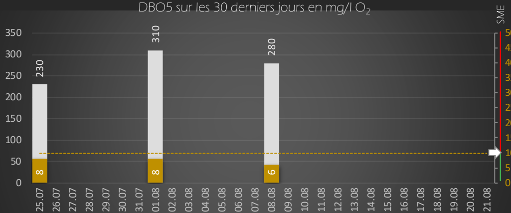
DBO5 sur les 30 derniers jours en mg/l O 2
